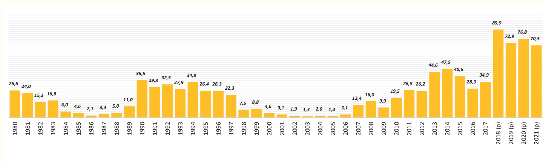
GRÁFICO N° 61: VALOR DE PRODUCCIÓN DE MINERALES: COCHABAMBA (En Miles de Dólares Americanos) Serie: 1980 - 2021
