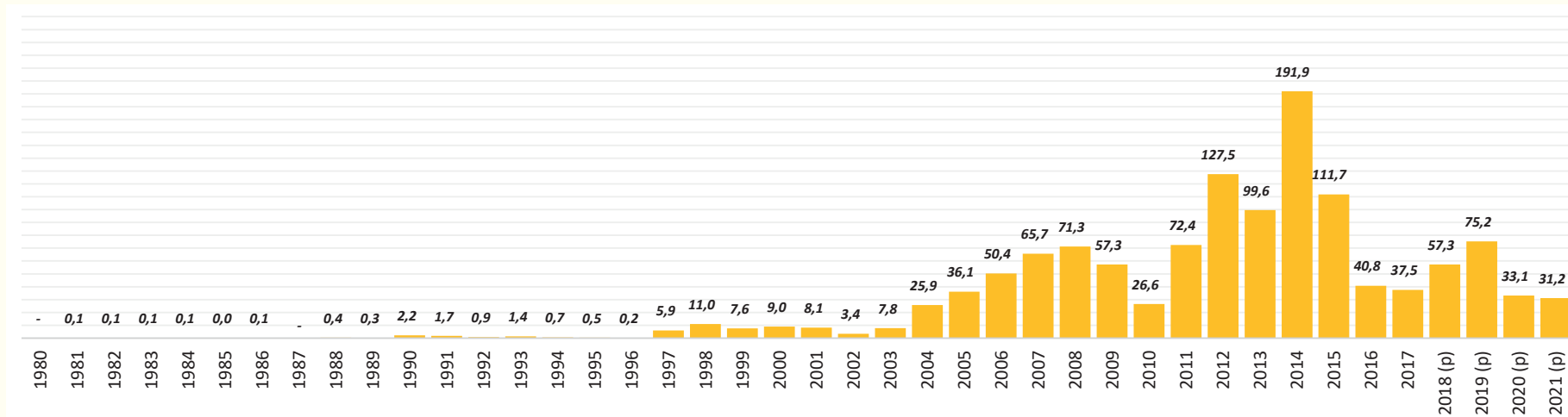
GRÁFICO N° 69: VALOR DE PRODUCCIÓN DE MINERALES: SANTA CRUZ (En Miles de Dólares Americanos) Serie: 1980 - 2021
