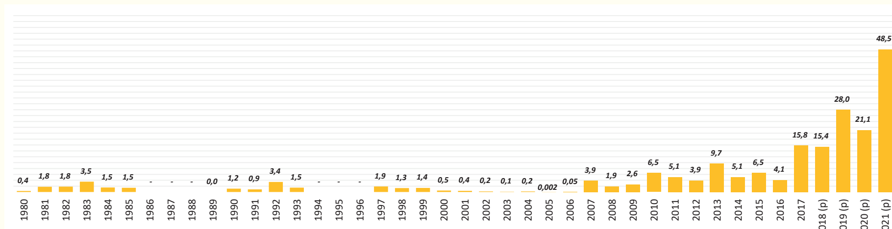
GRÁFICO N° 57: VALOR DE PRODUCCIÓN DE MINERALES: CHUQUISACA (En Miles de Dólares Americanos) Serie: 1980 - 2021
