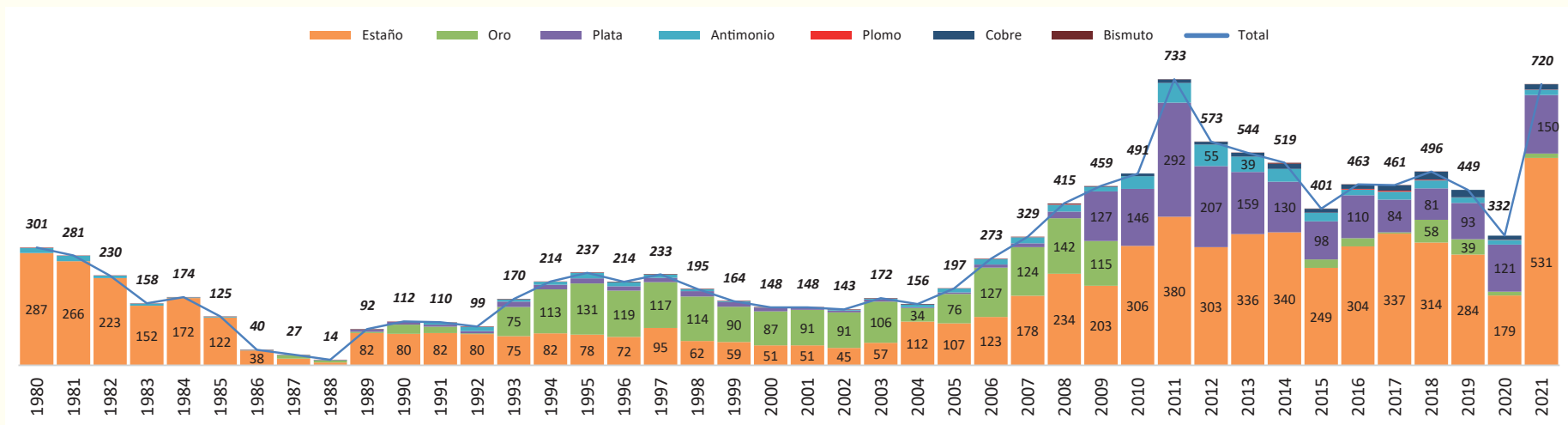
GRÁFICO N° 73: PRODUCCIÓN NACIONAL DE MINERALES METÁLICOS (En Millones de Dólares Americanos) Serie: 1980 - 2021
