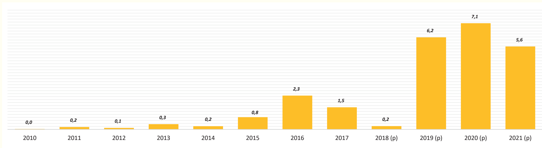
GRÁFICO N° 67: VALOR DE PRODUCCIÓN DE MINERALES: TARIJA (En Miles de Dólares Americanos) Serie: 2010 - 2021
