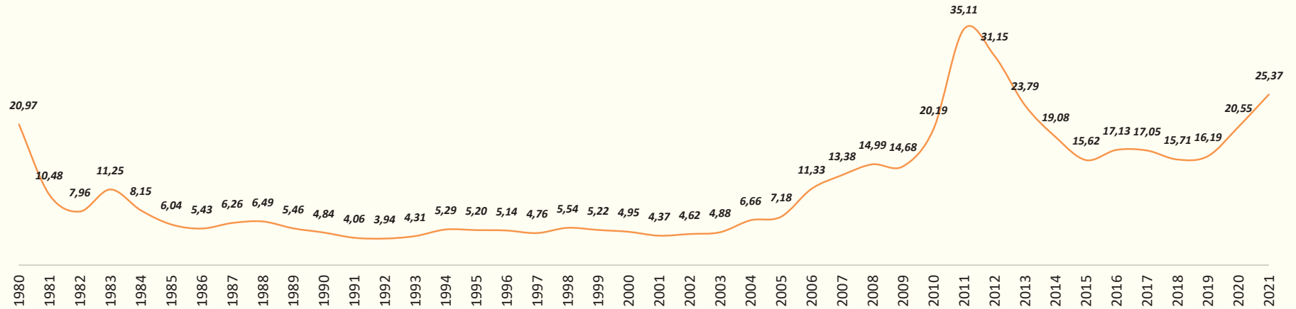
GRÁFICO 153: PRECIOS NOMINALES DE LA PLATA (EN DÓLARES AMERICANOS POR ONZA TROY) Serie: 1980 - 2021
