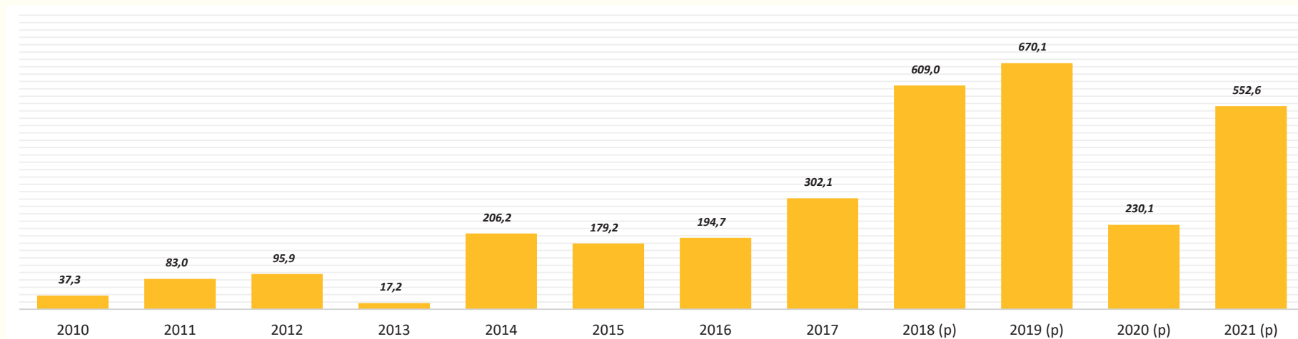
GRÁFICO N° 71: VALOR DE PRODUCCIÓN DE MINERALES: BENI (En Miles de Dólares Americanos) Serie: 2010 - 2021
