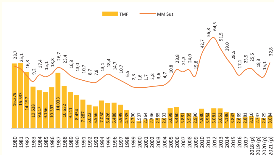
GRÁFICO N° 42: PRODUCCIÓN NACIONAL DE ANTIMONIO (En TMF y Millones de Dólares Americanos) Serie: 1980 - 2021
