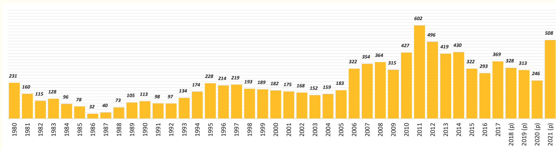
GRÁFICO N° 63: VALOR DE PRODUCCIÓN DE MINERALES: ORURO (En Miles de Dólares Americanos) Serie: 1980 - 2021
