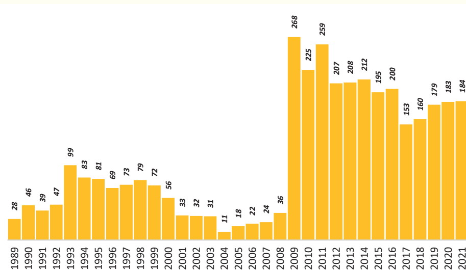
GRÁFICO N° 78: PRODUCCIÓN NACIONAL DE PLATA METÁLICA (En Toneladas Métricas Finas) Serie: 1980 - 2021
