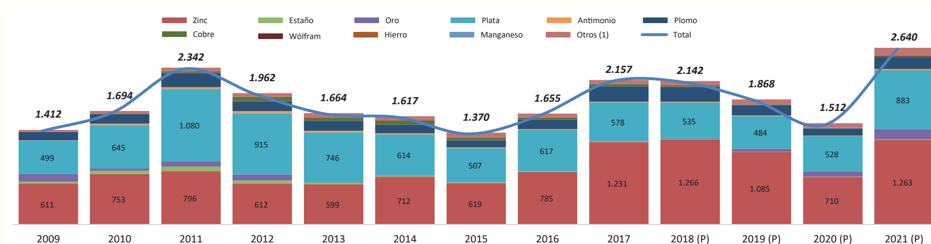
GRÁFICO N° 49: VALOR DE PRODUCCIÓN DE PRINCIPALES MINERALES DE LA MINERÍA PRIVADA (En Millones de Dólares Americanos) Serie: 2009 - 2021
