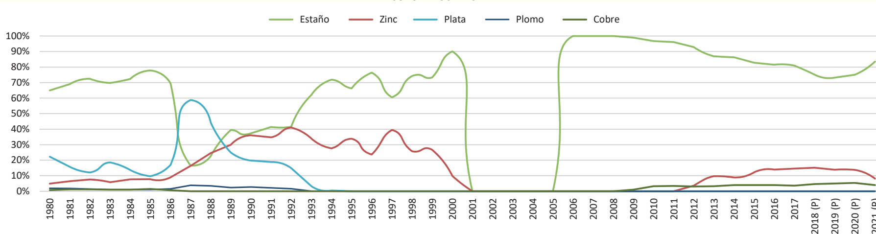
GRÁFICO N° 47: COMPOSICIÓN DEL VALOR DE PRODUCCIÓN DE PRINCIPALES MINERALES DE LA MINERÍA ESTATAL (En Porcentajes) Serie: 1980 - 2021
