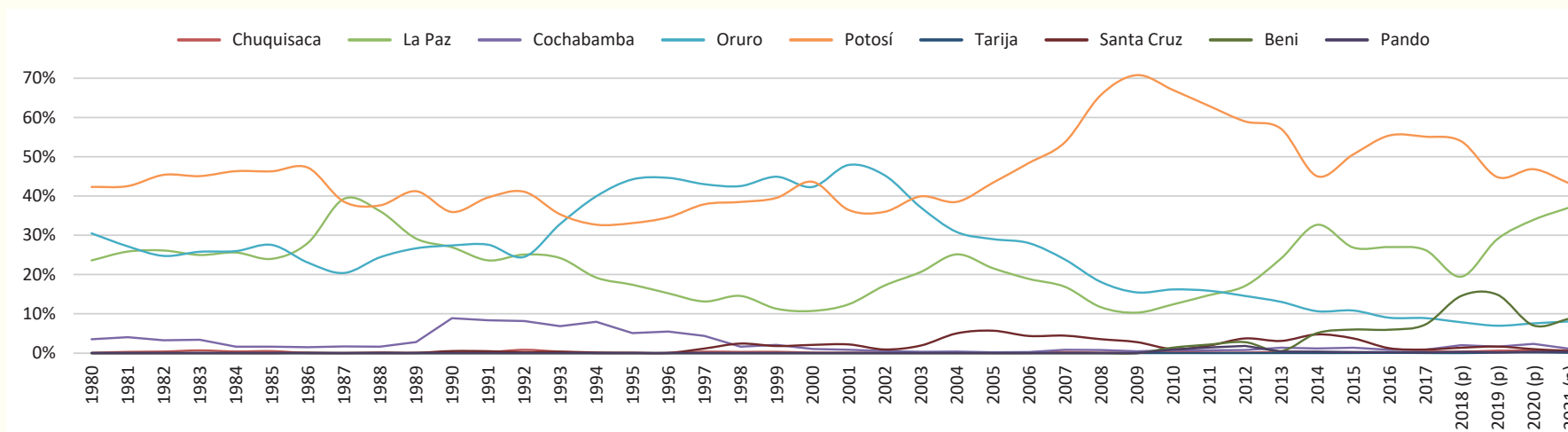
GRÁFICO N° 56: PARTICIPACIÓN POR DEPARTAMENTOS EN LA PRODUCCIÓN NACIONAL DE MINERALES (En Porcentaje) Serie: 1980 - 2021
