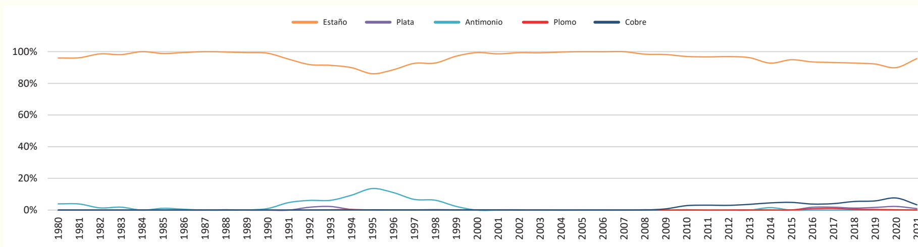
GRÁFICO N° 80: PRODUCCIÓN DE MINERALES METÁLICOS DE LA MINERÍA ESTATAL (En Porcentajes) Serie: 1980 - 2021
