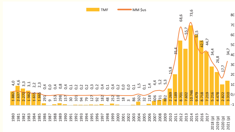
GRÁFICO N° 45: PRODUCCIÓN NACIONAL DE COBRE (En TMF y Millones de Dólares Americanos) Serie: 1980 - 2021
