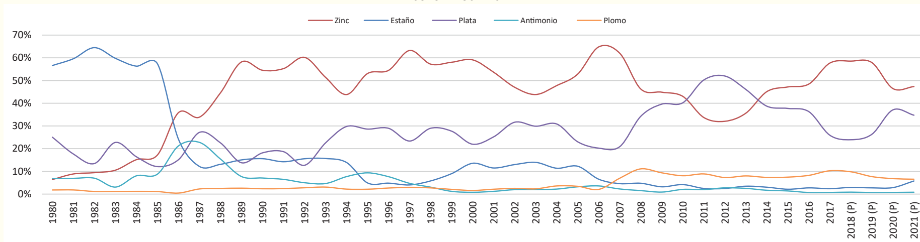
GRÁFICO N° 66: COMPOSICIÓN DEL VALOR DE PRODUCCIÓN POR MINERALES: POTOSÍ (En Porcentajes) Serie: 1980 - 2021
