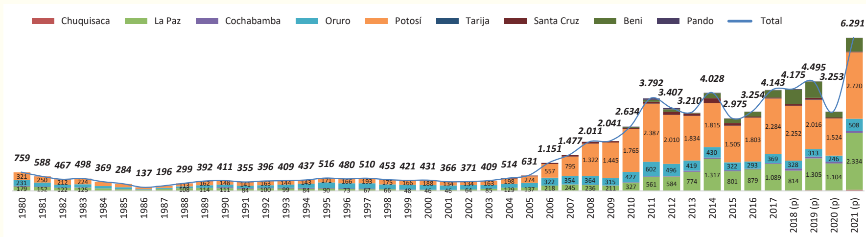
GRÁFICO N° 55: PRODUCCIÓN DE MINERALES POR DEPARTAMENTOS (En MM de Dólares Americanos) Serie: 1980 - 2021
