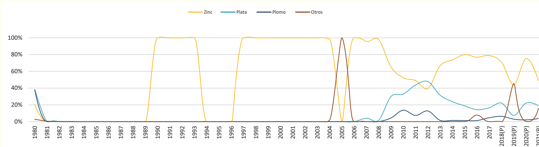
GRÁFICO N° 58: COMPOSICIÓN DEL VALOR DE PRODUCCIÓN POR MINERALES: CHUQUISACA (En Porcentajes) Serie: 1980 - 2021
