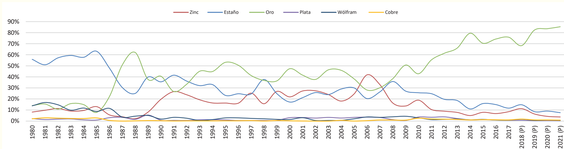
GRÁFICO N° 60: COMPOSICIÓN DEL VALOR DE PRODUCCIÓN POR MINERALES: LA PAZ (En Porcentajes) Serie: 1980 - 2021
