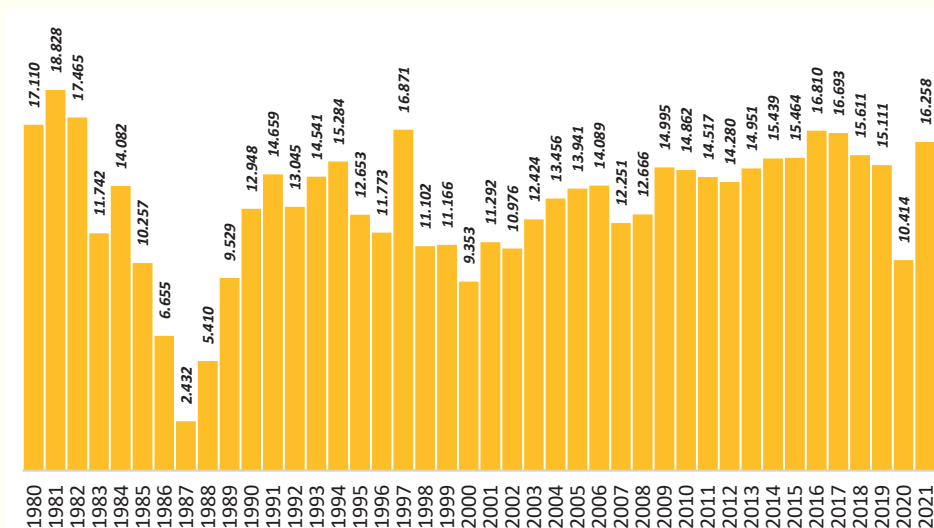
GRÁFICO N° 75: PRODUCCIÓN NACIONAL DE ESTAÑO METÁLICO (En Toneladas Métricas Finas) Serie: 1980 - 2021
