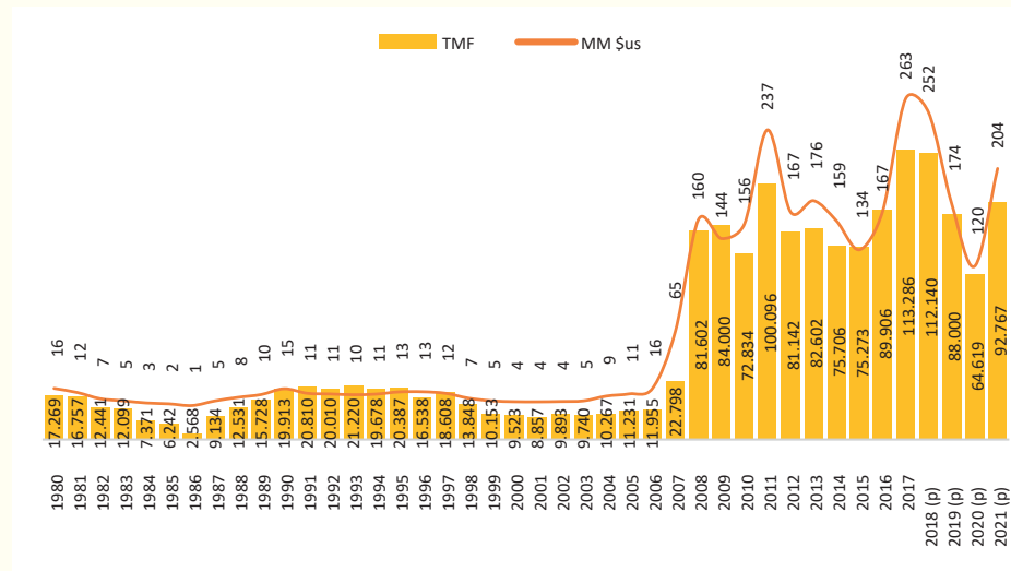
GRÁFICO N° 43: PRODUCCIÓN NACIONAL DE PLOMO (En TMF y Millones de Dólares Americanos) Serie: 1980 - 2021
