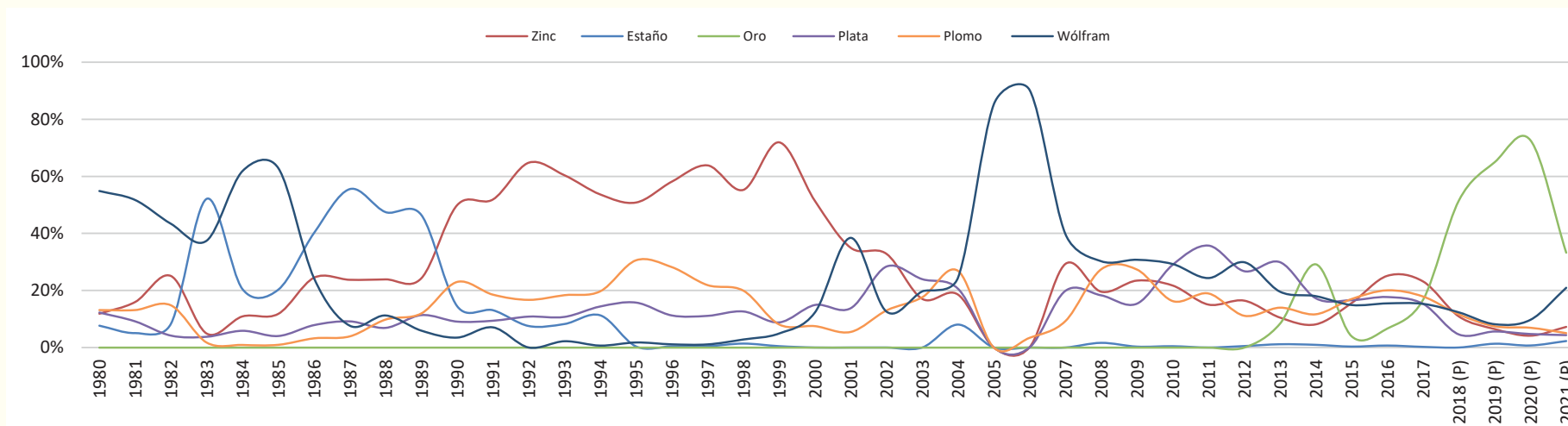
GRÁFICO N° 62: COMPOSICIÓN DEL VALOR DE PRODUCCIÓN POR MINERALES: COCHABAMBA (En Porcentajes) Serie: 1980 - 2021
