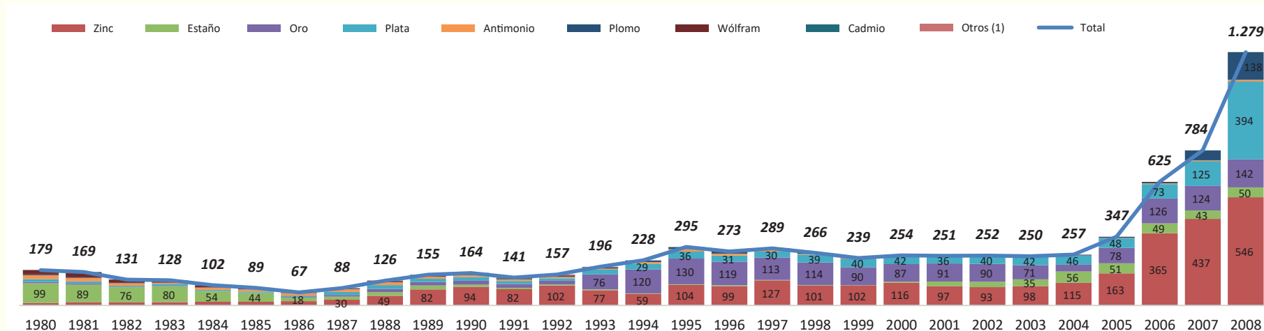
GRÁFICO N° 48: VALOR DE PRODUCCIÓN DE PRINCIPALES MINERALES DE LA MINERÍA MEDIANA (En Millones de Dólares Americanos) Serie: 1980 - 2008
