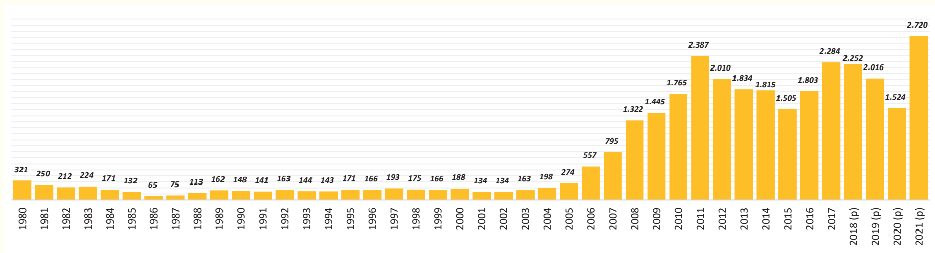
GRÁFICO N° 65: VALOR DE PRODUCCIÓN DE MINERALES: POTOSÍ (En Miles de Dólares Americanos) Serie: 1980 - 2021
