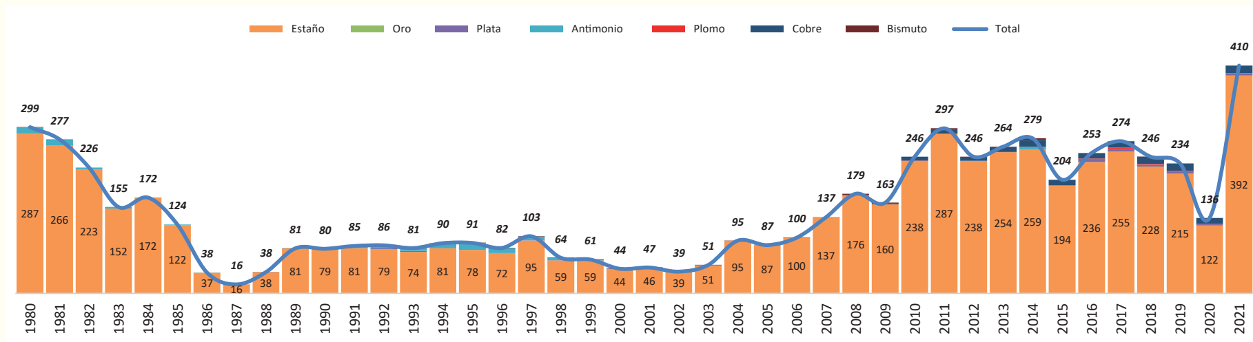
GRÁFICO N° 79: PRODUCCIÓN DE MINERALES METÁLICOS DE LA MINERÍA ESTATAL (En Millones de Dólares Americanos) Serie: 1980 - 2021
