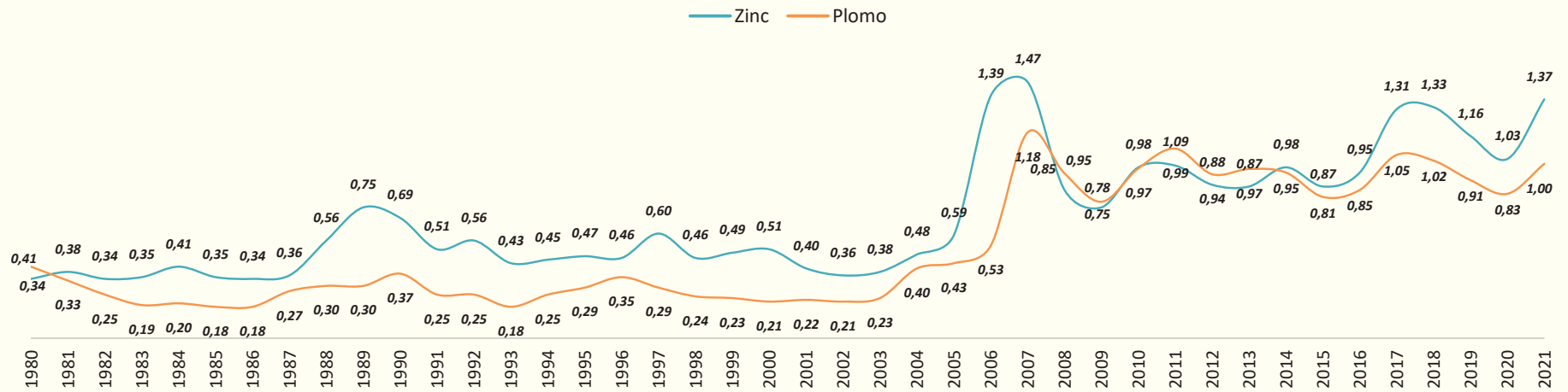
GRÁFICO 154: PRECIOS NOMINALES DEL ZINC Y PLOMO (EN DÓLARES AMERICANOS POR LIBRA FINA) Serie: 1980 - 2021
