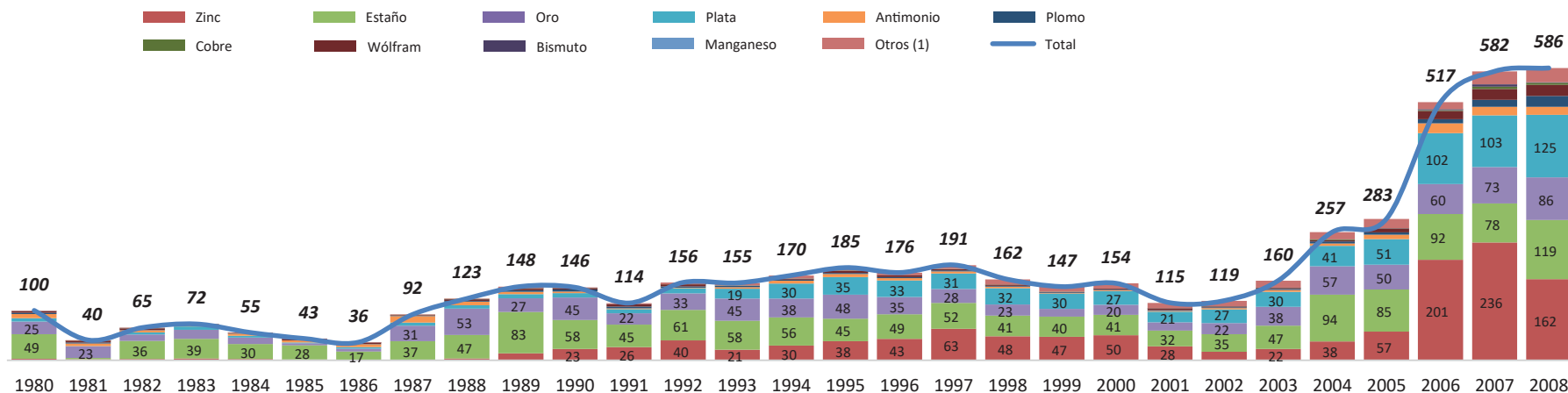
GRÁFICO N° 50: VALOR DE PRODUCCIÓN DE PRINCIPALES MINERALES DE MINERÍA CHICA Y LAS COOPERATIVAS (En Millones de Dólares Americanos) Serie: 1980 - 2008
