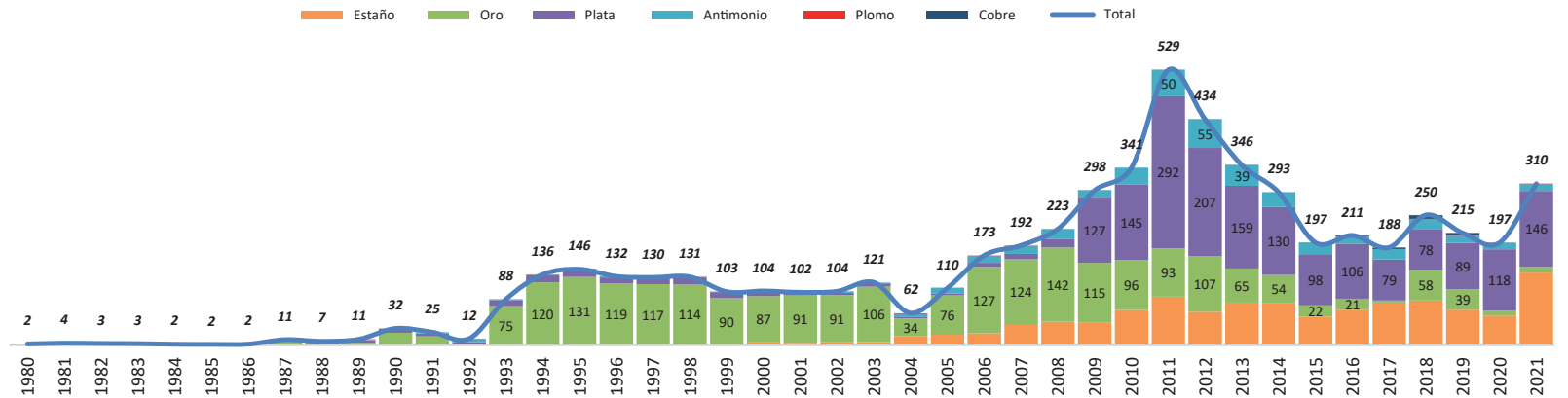
Viceministerio de Política Minera, Regulación y Fiscalización GRÁFICO N° 81: PRODUCCIÓN DE MINERALES METÁLICOS DE LA MINERÍA PRIVADA (En Millones de Dólares Americanos) Serie: 1980 - 2021
