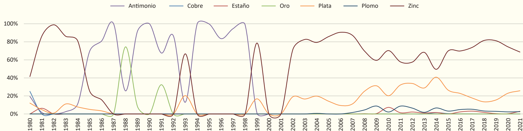
GRÁFICO N° 118: COMPOSICIÓN DE LA EXPORTACIÓN DE MINERALES A JAPÓN (En Porcentajes) Serie:1980 - 2021
