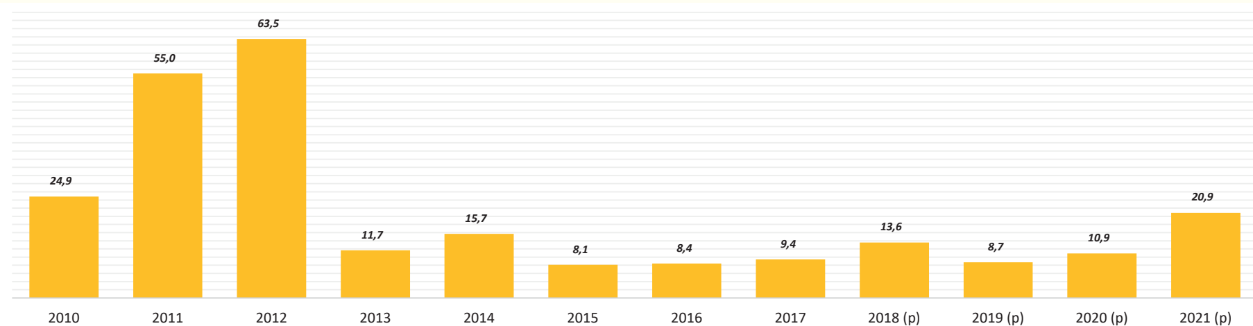
GRÁFICO N° 72: VALOR DE PRODUCCIÓN DE MINERALES: PANDO (En Miles de Dólares Americanos) Serie: 2010 - 2021
