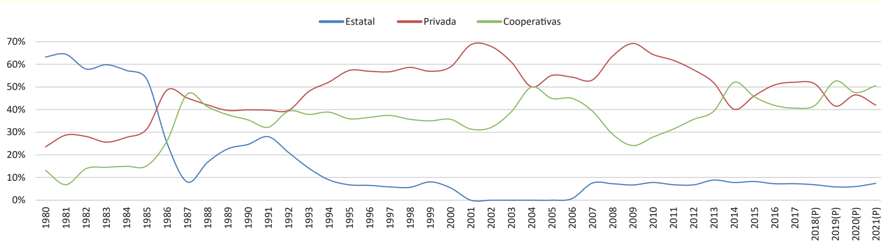
GRÁFICO N° 54: PARTICIPACIÓN EN VALOR DE PRODUCCIÓN DE MINERALES POR ACTOR PRODUCTIVO MINERO (En Porcentajes) Serie: 1980 - 2021
