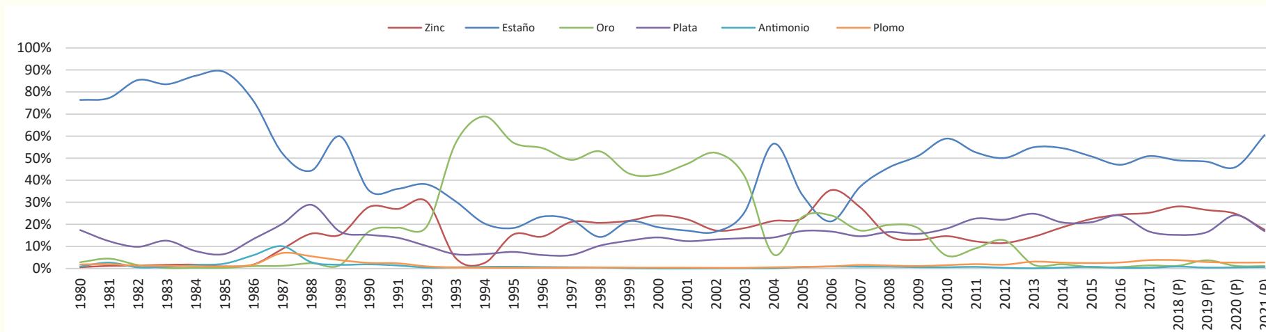
GRÁFICO N° 64: COMPOSICIÓN DEL VALOR DE PRODUCCIÓN POR MINERALES: ORURO (En Porcentajes) Serie: 1980 - 2021
