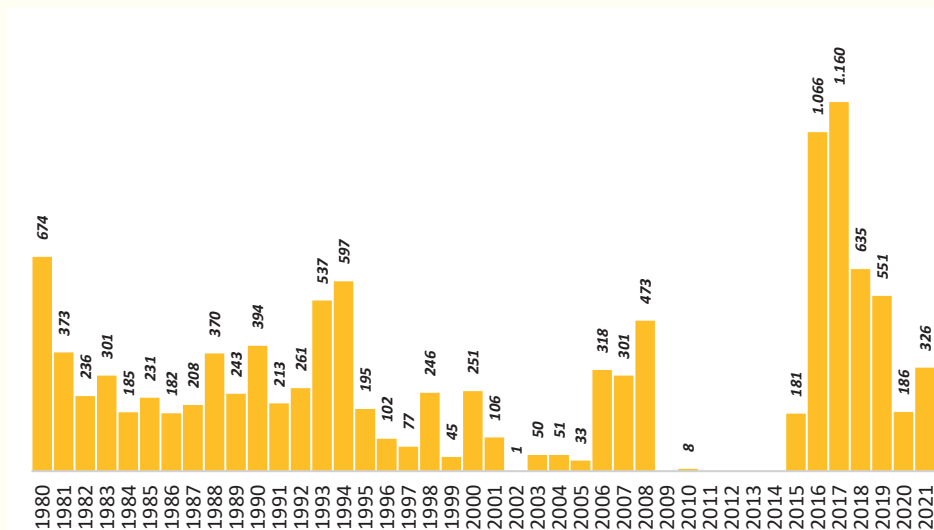
GRÁFICO N° 77: PRODUCCIÓN NACIONAL DE PLOMO METÁLICO (En Toneladas Métricas Finas) Serie: 1980 - 2021
