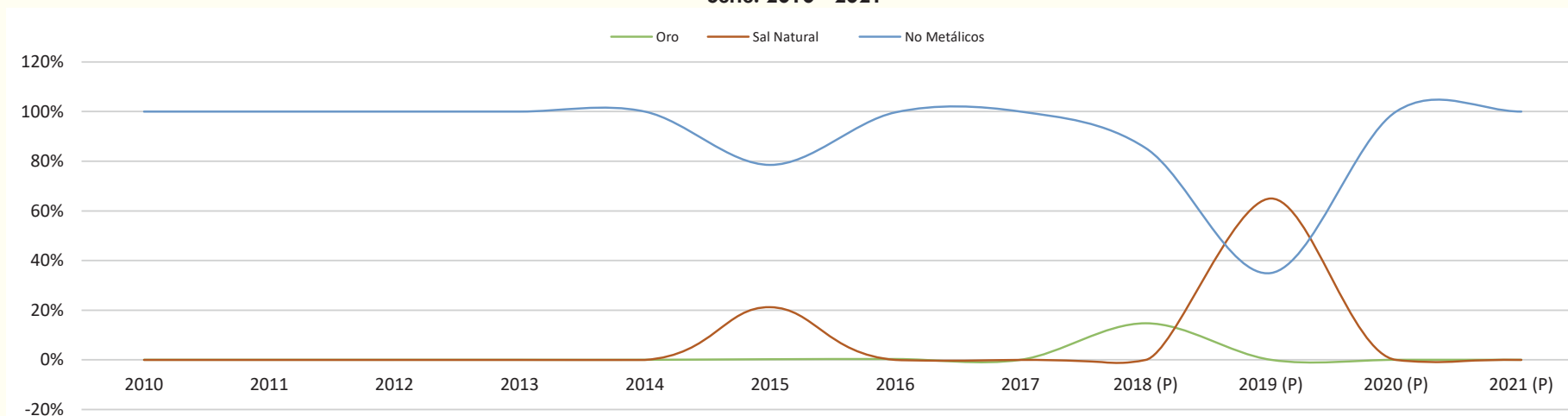
GRÁFICO N° 68: COMPOSICIÓN DEL VALOR DE PRODUCCIÓN POR MINERALES: TARIJA (En Porcentajes) Serie: 2010 - 2021
