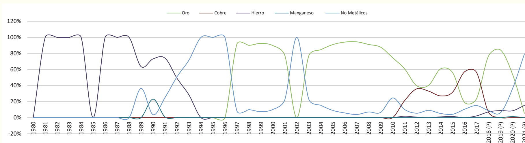
GRÁFICO N° 70: COMPOSICIÓN DEL VALOR DE PRODUCCIÓN POR MINERALES: SANTA CRUZ (En Porcentajes) Serie: 1980 - 2021
