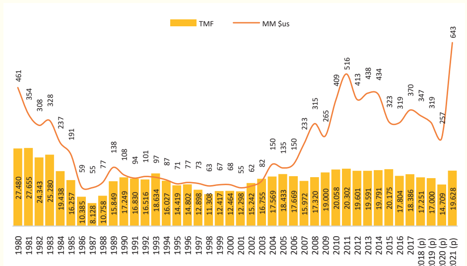
GRÁFICO N° 39: PRODUCCIÓN NACIONAL DE ESTAÑO (En TMF y Millones de Dólares Americanos) Serie: 1980 - 2021
