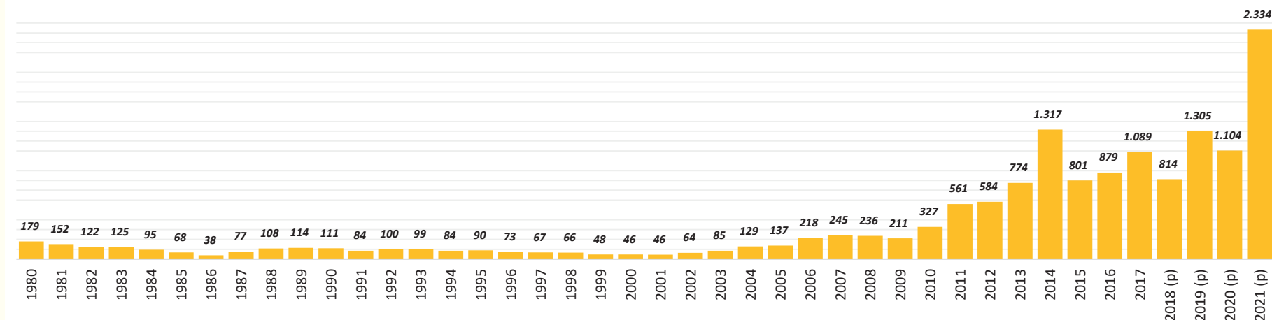
GRÁFICO N° 59: VALOR DE PRODUCCIÓN DE MINERALES: LA PAZ (En Miles de Dólares Americanos) Serie: 1980 - 2021
