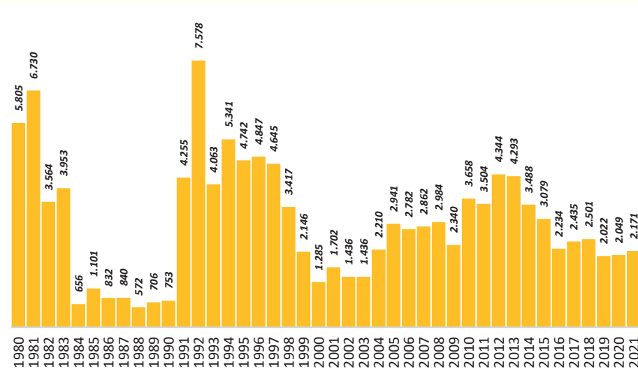
GRÁFICO N° 76: PRODUCCIÓN NACIONAL DE ANTIMONIO METÁLICO (En Toneladas Métricas Finas) Serie: 1980 - 2021
