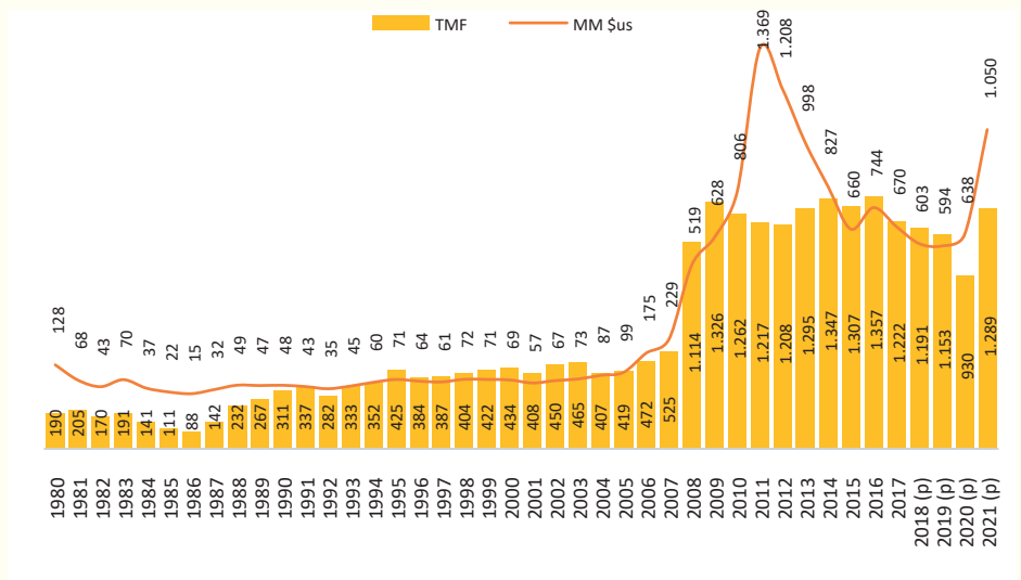
GRÁFICO N° 41: PRODUCCIÓN NACIONAL DE PLATA (En TMF y Millones de Dólares Americanos) Serie: 1980 - 2021
