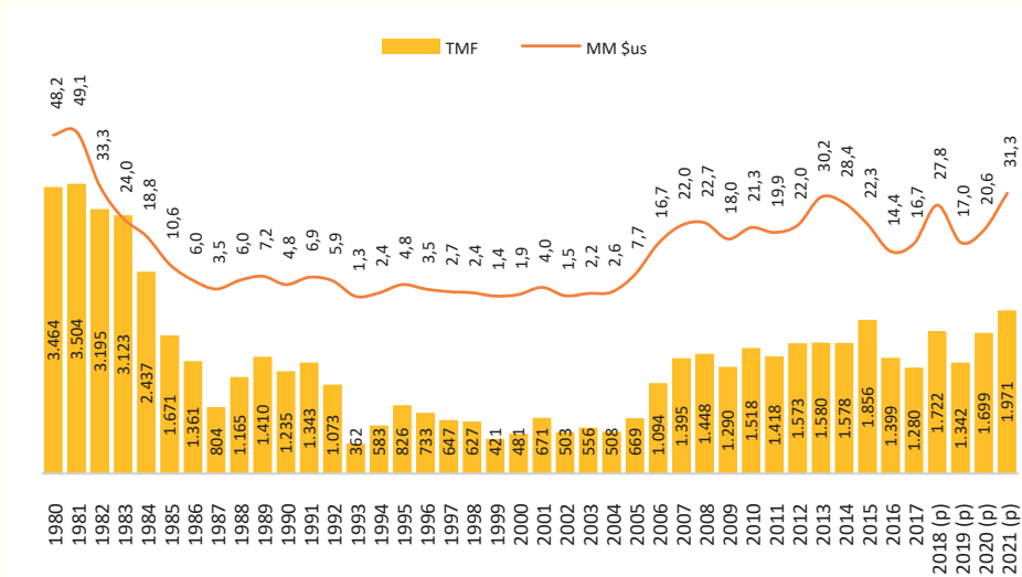
GRÁFICO N° 44: PRODUCCIÓN NACIONAL DE WÓLFRAM (En TMF y Millones de Dólares Americanos) Serie: 1980 - 2021
