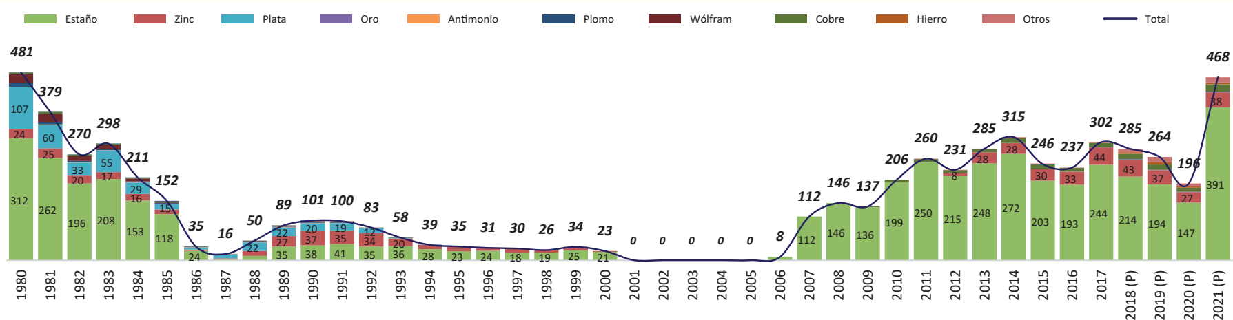
GRÁFICO N° 46: VALOR DE PRODUCCIÓN DE PRINCIPALES MINERALES DE LA MINERÍA ESTATAL (En Millones de Dólares Americanos) Serie: 1980 - 2021
