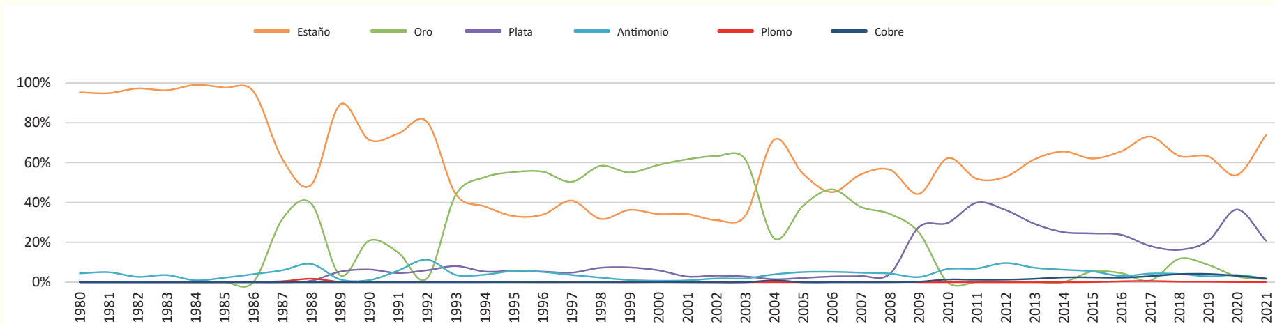
GRÁFICO N° 74: PARTICIPACIÓN EN LA PRODUCCIÓN NACIONAL DE MINERALES METÁLICOS (En Porcentajes) Serie: 1980 - 2021
