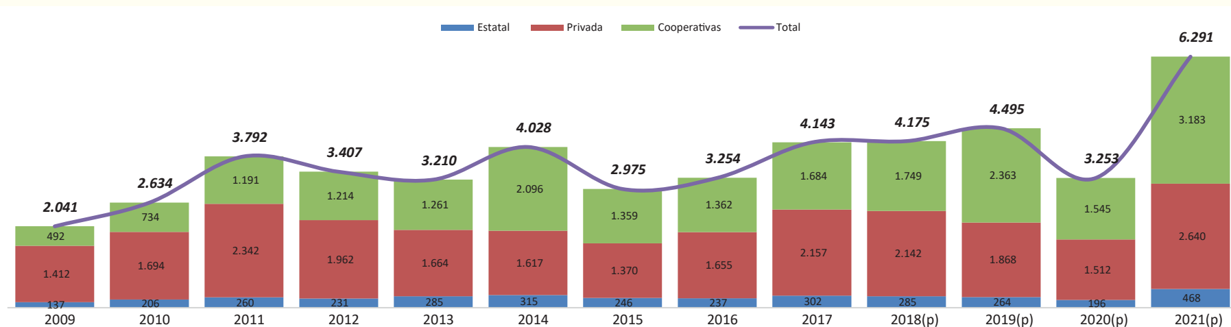
GRÁFICO N° 53: VALOR DE PRODUCCIÓN DE MINERALES POR ACTOR PRODUCTIVO MINERO (En MM de Dólares Americanos) Serie: 2009 - 2021
