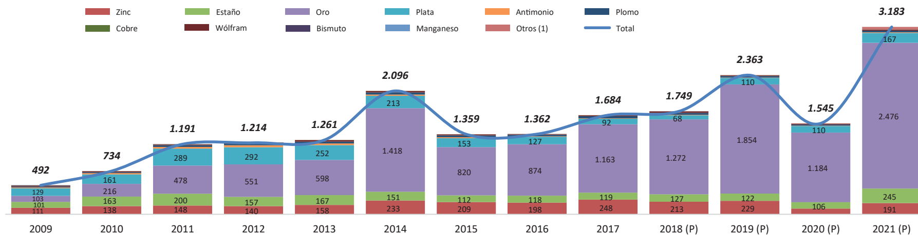
GRÁFICO N° 51: VALOR DE PRODUCCIÓN DE PRINCIPALES MINERALES DE LAS COOPERATIVAS (En Millones de Dólares Americanos) Serie: 2009 - 2021
