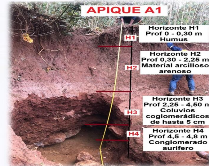
Perfil Apique A1. Sector Secundario
